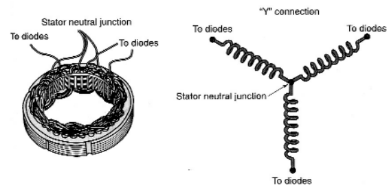
Y Connection
